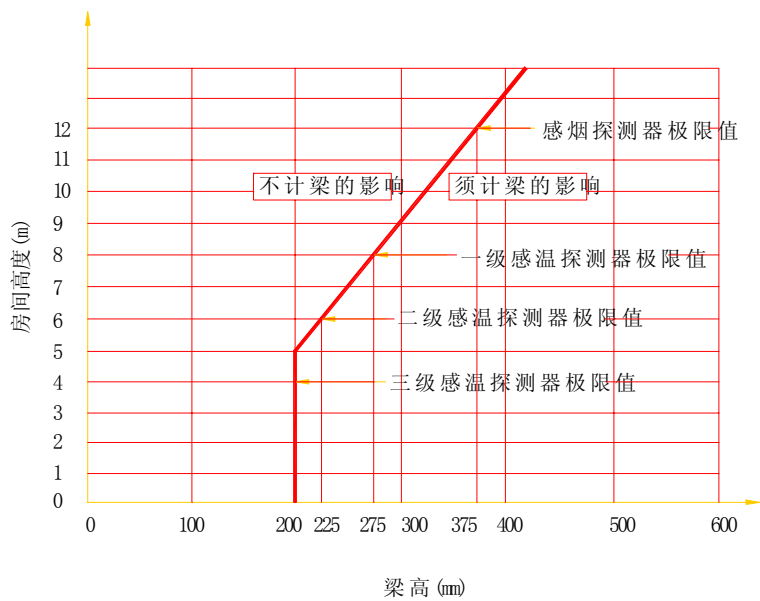
图 B 不同高度的房间梁对探测器设置的影响
