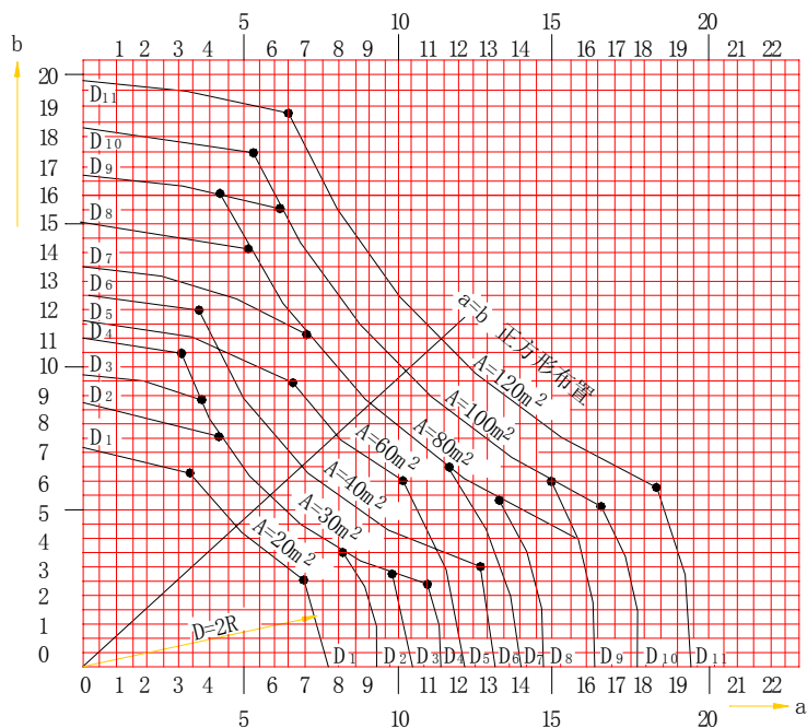
图 A 探测器安装间距的极限曲线
